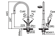
OLTEN TA9531B - 2264953
