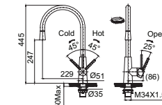
OLTEN TA9531 - 2003899
