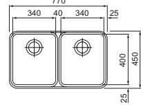
ANCONA ANX 120
