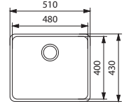
ANCONA ANX 110-48
