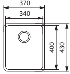
ANCONA ANX 110-34
