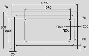
Domaine Inset Bath
