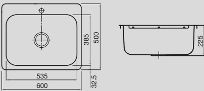
Domaine 45 Litre Laundry Trough
